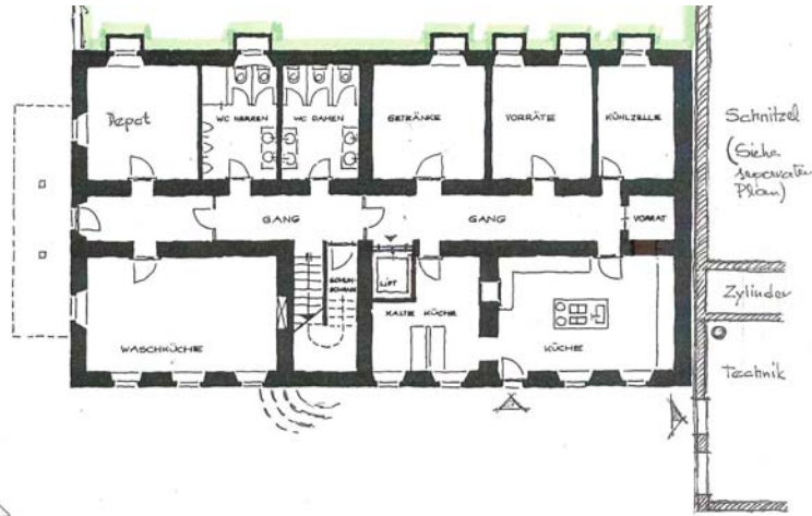
UNTERGESCHOSS
